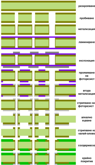
ПРИМЕРНА СХЕМА НА 4-СЛОЙНА ПЕЧАТНА ПЛАТКА
